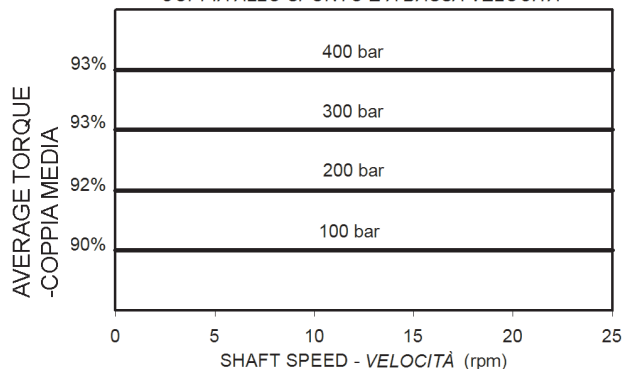
STARTING AND LOW SPEED TORQUE COPPIA ALLO SPUNTO E A BASSA VELOCITÀ
